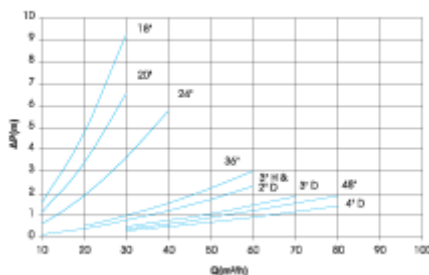
Diagramme: débit / pression
