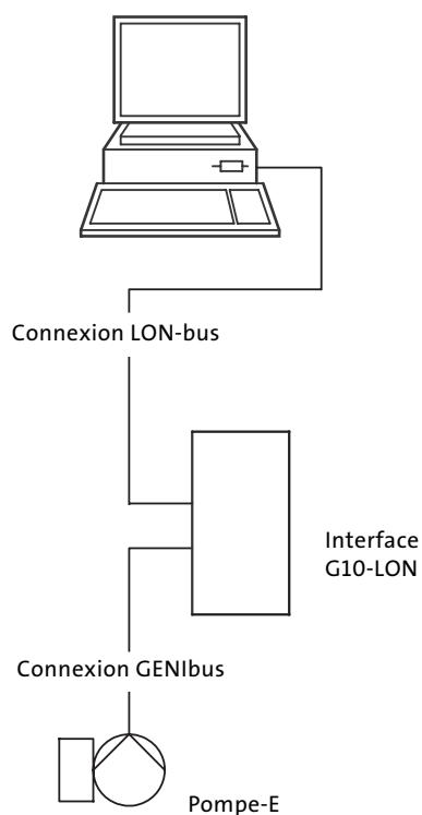
Fig. 6 Structure d'un poste central de télégestion
