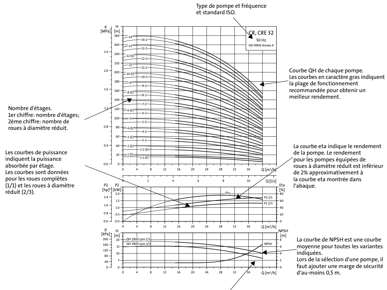
Courbe QH par étage. Les courbes pour les roues complètes (1/1) et les roues à diamètre réduit (2/3) sont indiquées.
