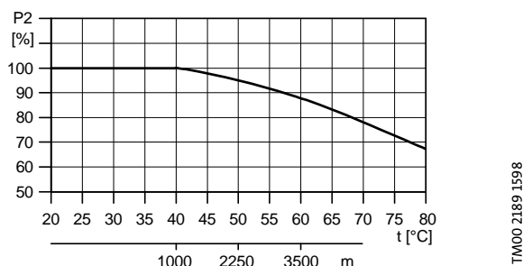
Fig. 5 Relation entre la puissance moteur (P2) et la température ambiante.
