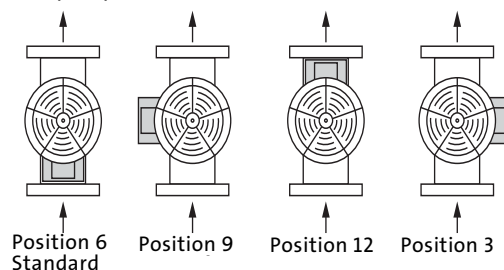
Fig. 4 Positions de la boîte à bornes
