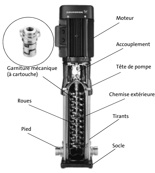
Fig. 3 Pompe CR
