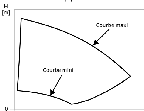
Fig. 19 Courbes de performances mini et maxi
