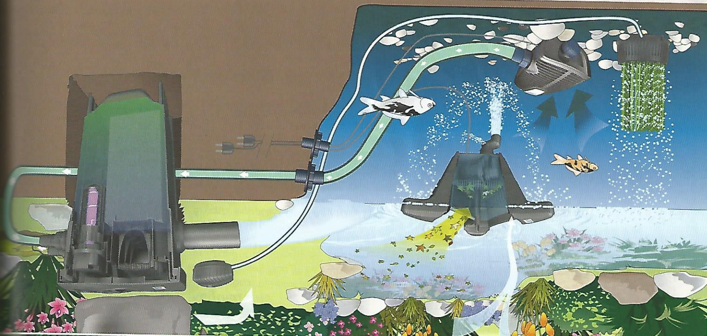
Représentation schématique : coordination des différents composants du système Clear Water System
